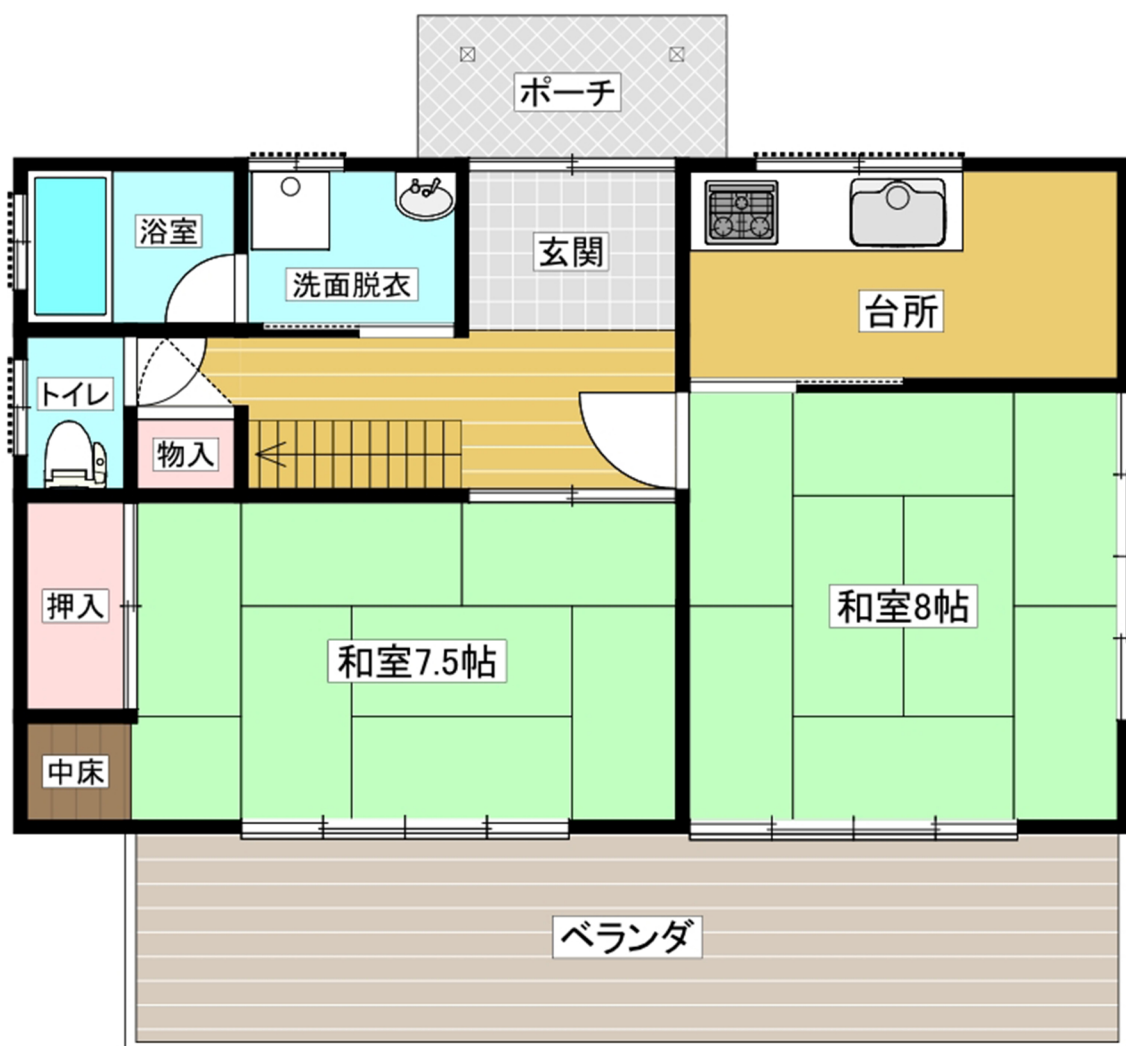
1階 間取図
