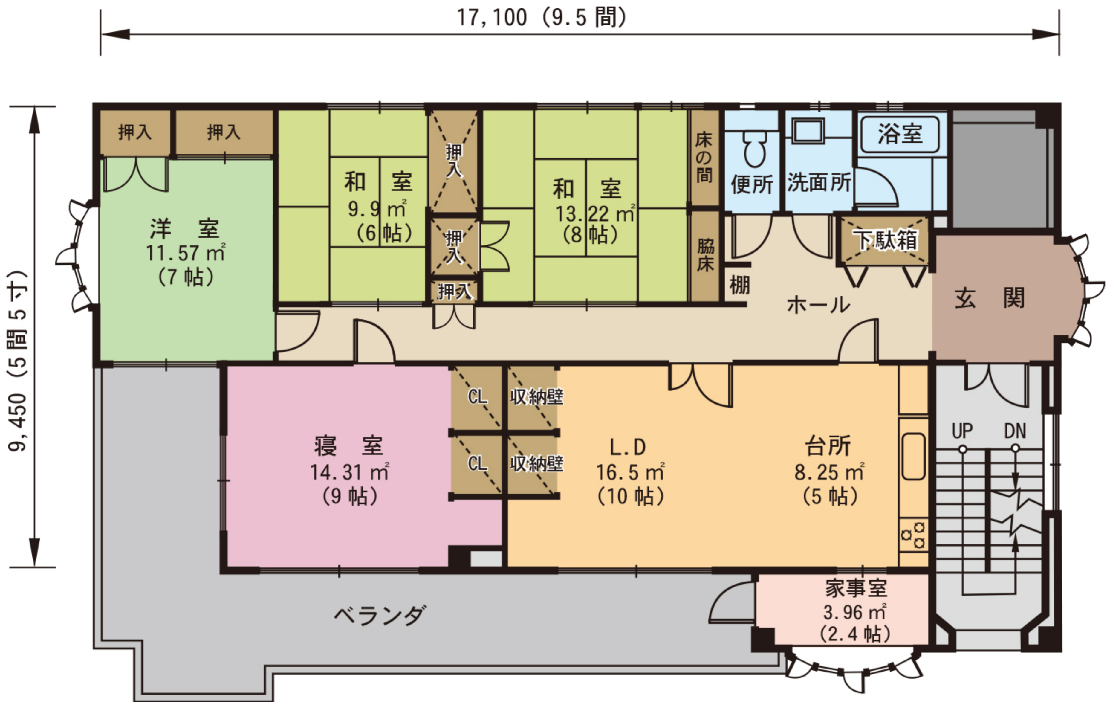
3 階平面図 床面積 137.83 m 2 (41.8 坪)
