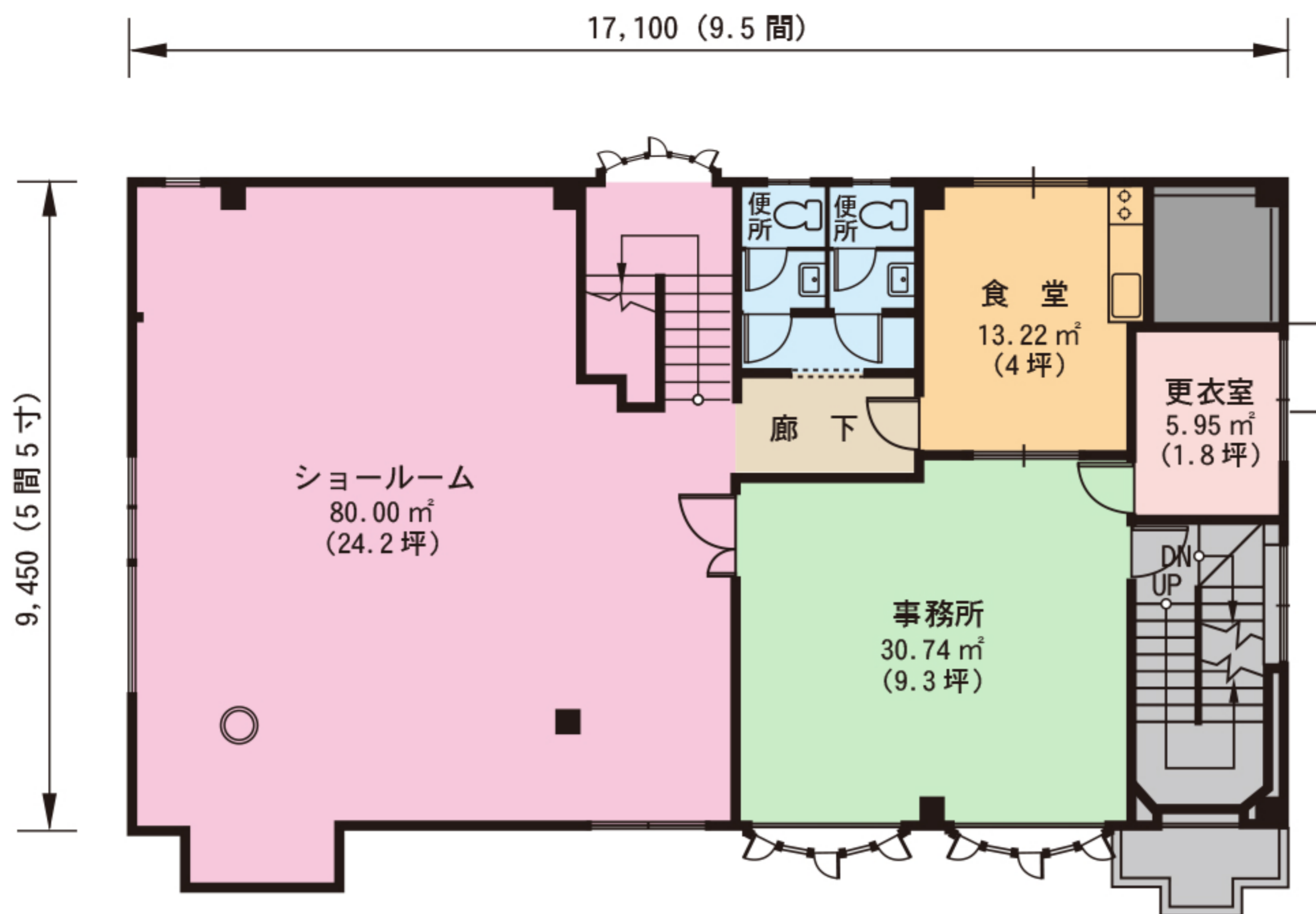
2 階平面図 床面積 163.36 m 2 (49.5 坪)
